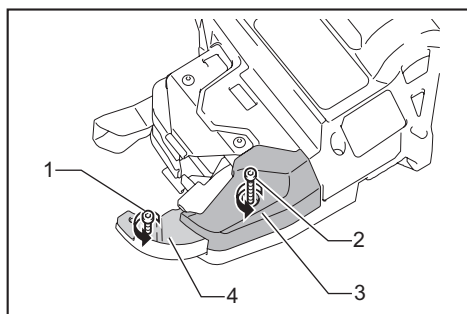
► 1. Boulon A 2. Boulon B 3. Couvercle de la plaque de contact 4. Guide-fil B
