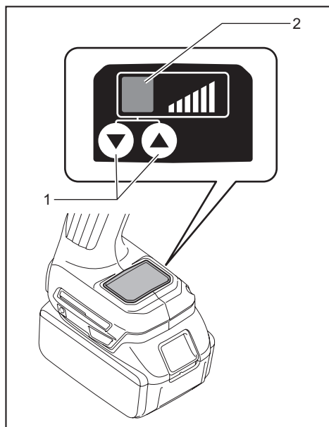
► 1. Bouton de réglage de la force de ligature 2. Panneau d'affichage
