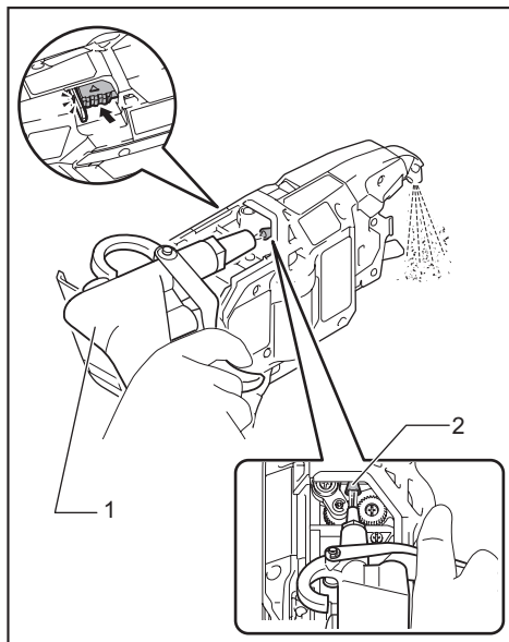
► 1. Pistolet à air comprimé 2. Guide
