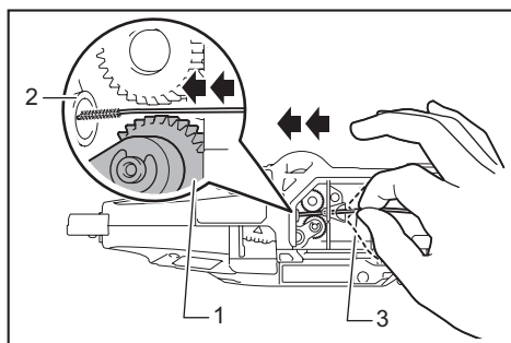
► 1. Roue 2. Guide 3. Brosse métallique
