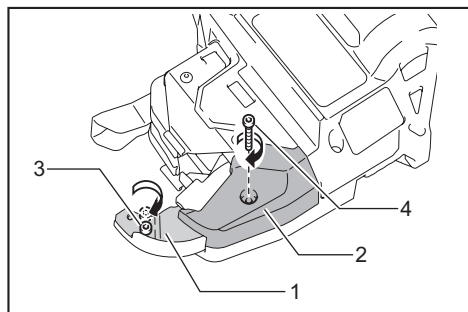
► 1. Guide-fil B 2. Couvercle de la plaque de contact 3. Boulon A 4. Boulon B
