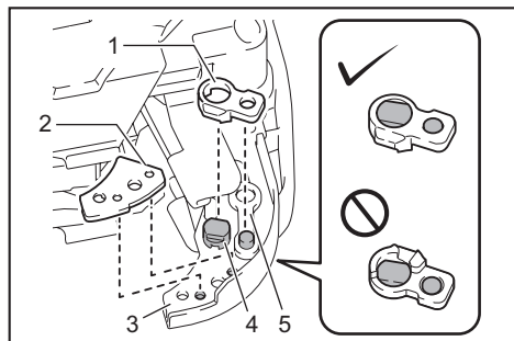
► 1. Coupe-fil B 2. Plaque supérieure 3. Plaque de bras A 4. Coupe-fil A 5. Bras de liaison A
