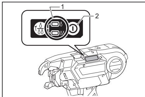
► 1. Témoin du mode de ligature 2. Bouton d'alimentation
