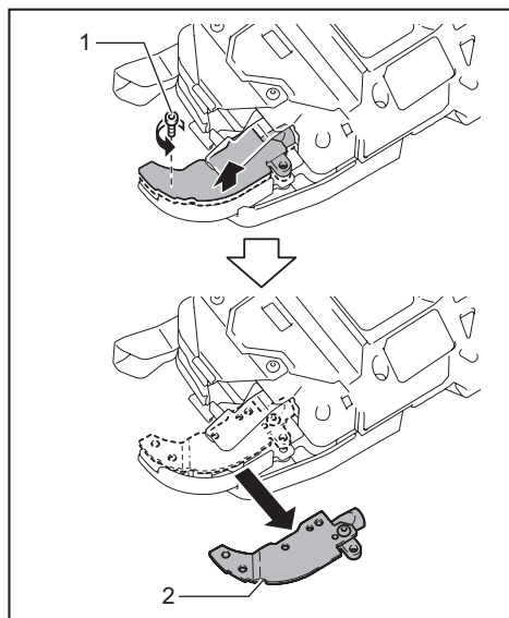
► 1. Boulon A 2. Guide-fil B
