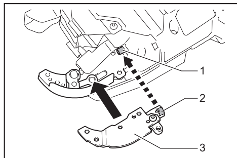
► 1. Tige 2. Rainure 3. Guide-fil B
