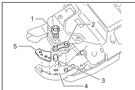
► 1. Cortadora B 2. Brazo articulado A 3. Cortadora A 4. Placa de brazo A 5. Placa superior
