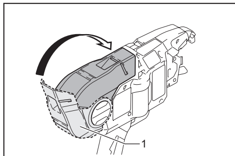
► 1. Couvercle de la bobine de fil
