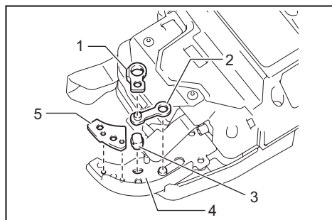
► 1. Coupe-fil B 2. Bras de liaison A 3. Coupe-fil A 4. Plaque de bras A 5. Plaque supérieure
